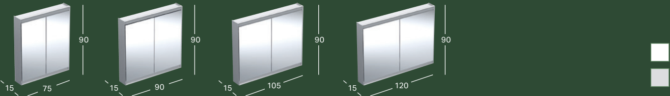
GEBERIT ONE SPEJLSKAB MED COMFORTLIGHT OG TO LÅGER, SYNLIG VÆGMONTERING, HØJDE 90 CM
