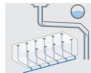
Konventionelt tagafvandingssystem
