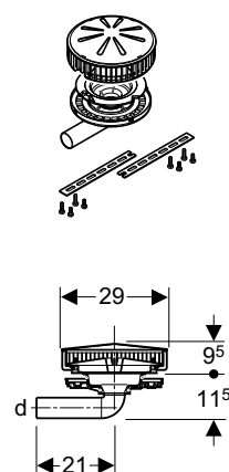
Pluvia tagbrønd med vandret afgang Geberit-nr. 359.565.00.1 VWS nr. 153732.056
