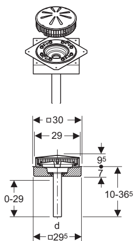
Pluvia tagbrønd Geberit-nr. 359.003.00.1 VWS nr. 153753.056
