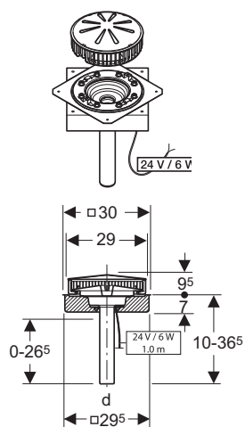
Pluvia tagbrønd med frostsikring Geberit-nr. 359.004.00.1 VWS nr. 153754.056
