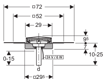
Pluvia tagbrønd med formonteret tagpap og inkl. frostsikring Geberit nr. 350.030.00.1 VVS nr. 153752.356
