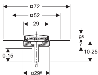
Pluvia tagbrønd med formonteret tagpap Geberit nr. 350.029.00.1 VVS nr. 153751.356
